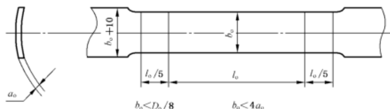
图 3 拉伸试样图
