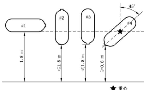
图7 跌落方向
