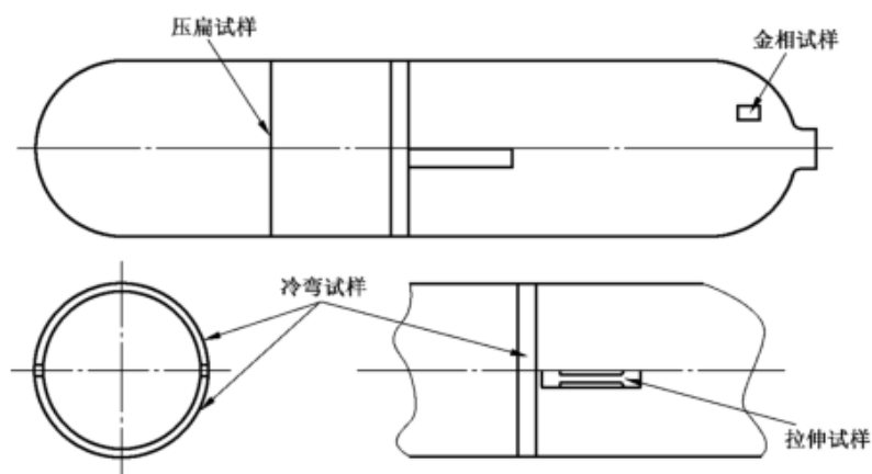
图 2 取样部位图
