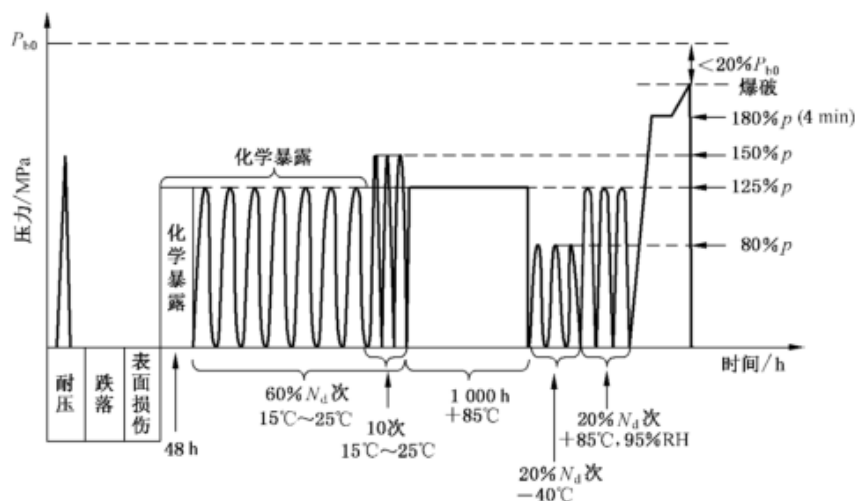
图 8 耐久性试验
